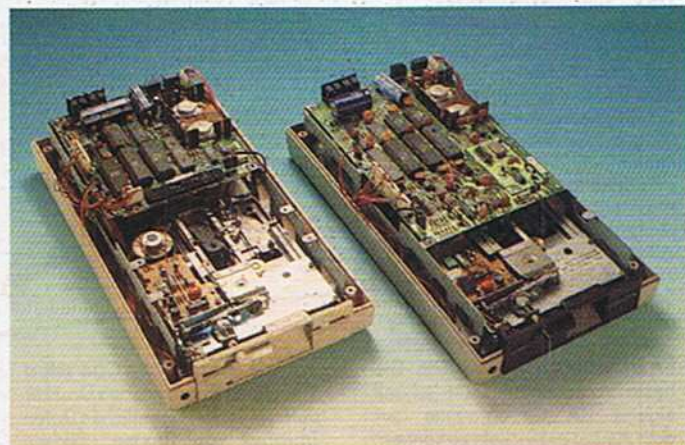
Bild 1. Ähnlich, aber nicht gleich: 1541 mal zwei
