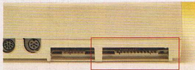
Bild 3. Der User-Port des C 64
