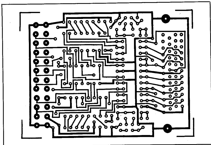
Bild 3a. Das Layout für die Schnittstelle (spiegelverkehrt)
