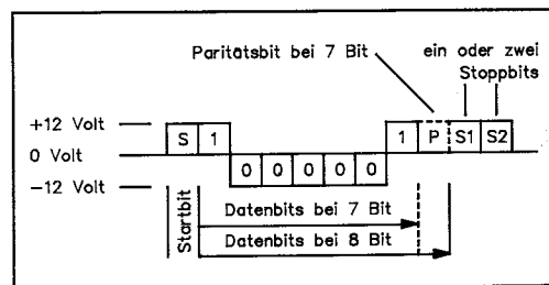
Bild 2. Format eines seriellen Datenwortes. Ein Start-Bit, 7 oder 8 Datenbit, ein Paritätsbit (bei 7 Datenbit)
