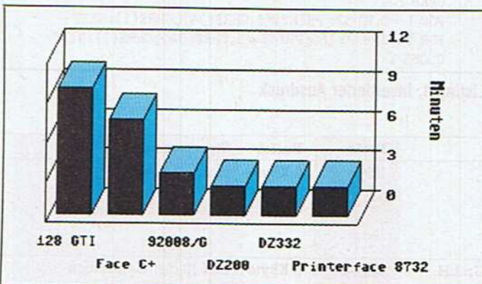
Bild 8. Zeitbedarf für den Ausdruck einer HiRes-Grafik
