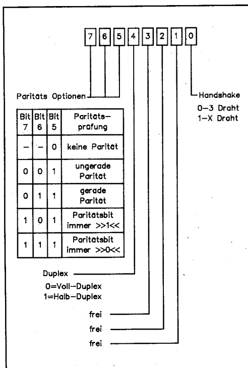
Bild 6. Das Befehlsregister dient mit seinen vollen 8 Bit der zusätzlichen Konfiguration der RS232C
