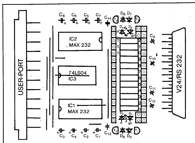
Bild 3b. Der Bestückungsplan für das RS232-Interface
