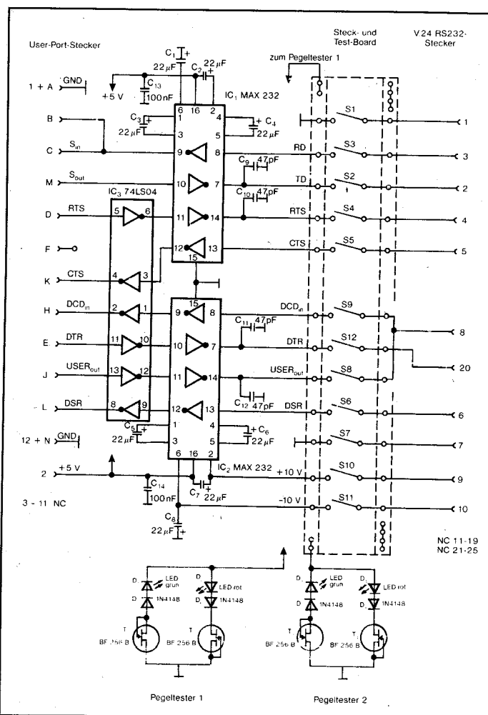
Bild 2. Der Schaltplan für die RS232-Schnittstelle
