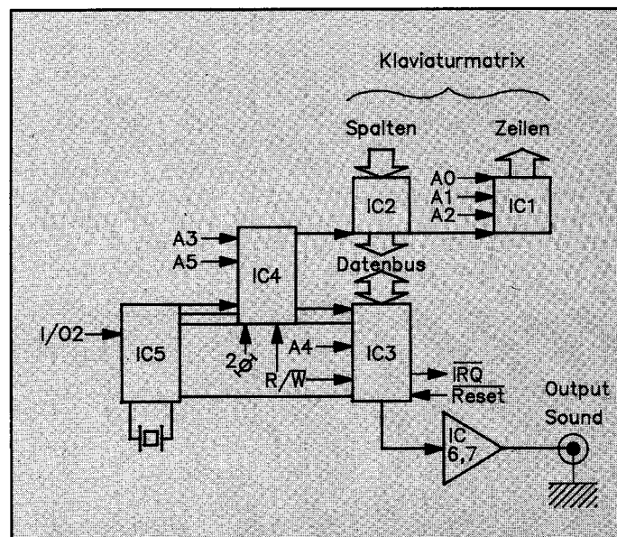
Bild 3. Blockschahtbild des SFX-Moduls
