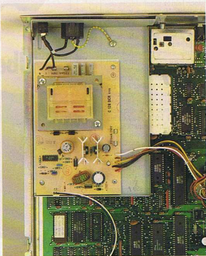
Bild 3. Das »nackte« Netzteil des neuen C 128D im Detail
