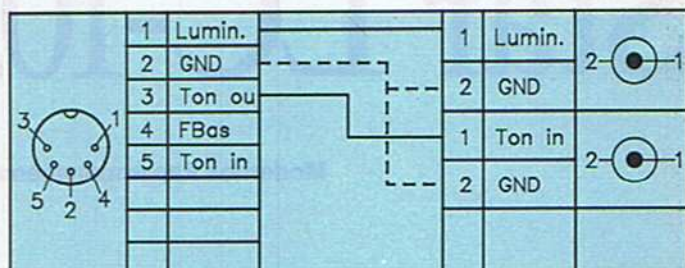
Bild 2. So schließt man einen monochromen Monitor an den C 64 oder C 128 an (gilt nur für 40-Zeichen-Bildschirm)
