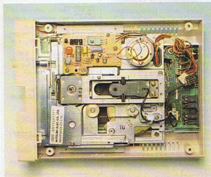
Bild 2. Das aufgeräumte Innenleben der 1541 II
