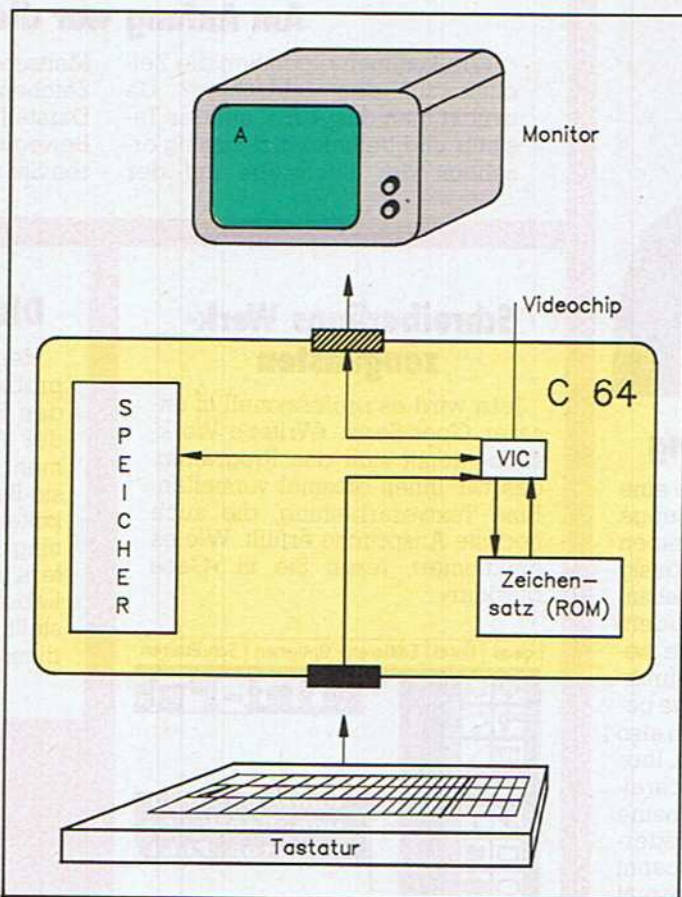
Bild 1. Schematisch zeigt diese Grafik den Weg von der Eingabe eines Zeichens über die Tastatur bis zur Darstellung auf dem Monitor. Nach dem Drücken der Taste legt der VIC den Wert im Speicher ab. Aus dem Zeichensatz wird die 8 x 8-Matrix für dieses Zeichen geholt und an den Monitor übermittelt.
