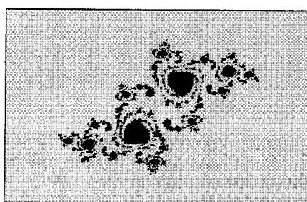
Bild 5. Eine Cantor-Menge für c = -0,194 + 0,6557i
