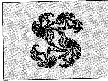
Bild 9. Der fraktale Kreis wird durch geringe Änderung des Wertes c in einen parabolischen Fall verwandelt
