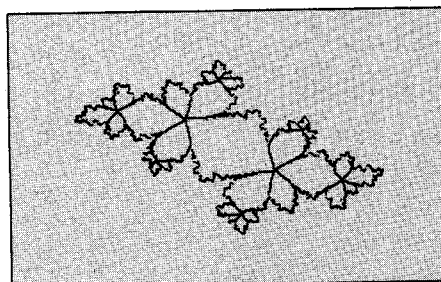
Bild 3. Parabolisches Basin um einen Fixpunkt für c = -0,481762 + 0,531657i
