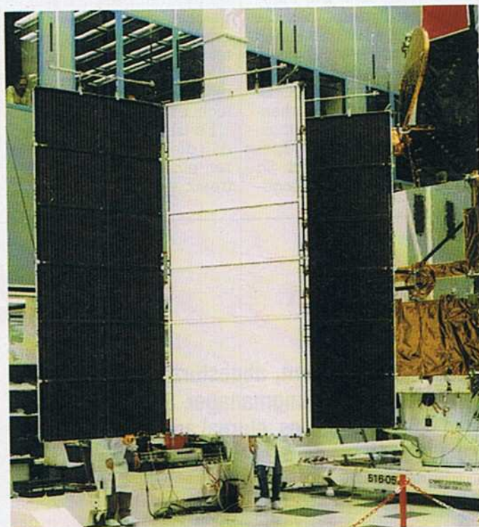
Bild 3. Der Solargenerator des TV-SAT 1 beim Entfalt-Test. Die einzelnen Flügel sind an einem Entfallsimulator aufgehängt.
