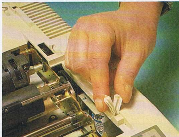
Bild 5. Der Sicherheitsschalter der Abdeckhaube muß überlistet werden
