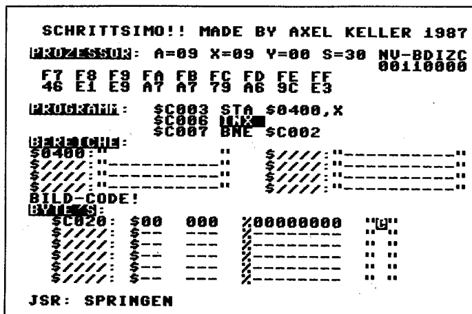
Bild 1. Mit der Simulatormaske lassen sich neben den Registern die Inhalte frei definierbarer Speicherbereiche und einzelner Bytes beobachten.
