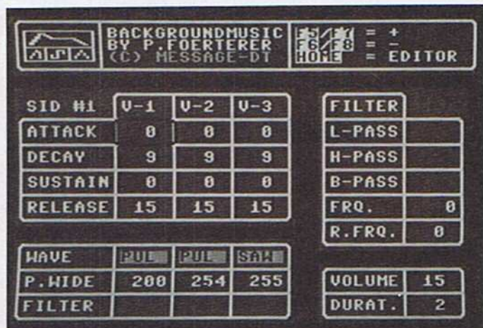
Die »Schaltzentrale« des Background Music Editors
