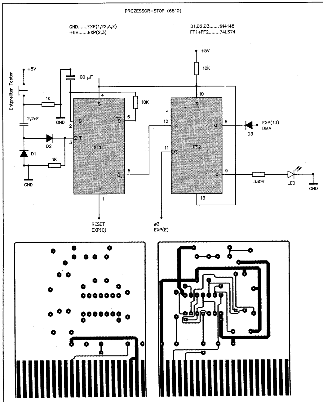
Layout (spiegelverkehrt), Bestückungsplan, Bauteileliste und Schaltbild zum »Prozessorstopp«
