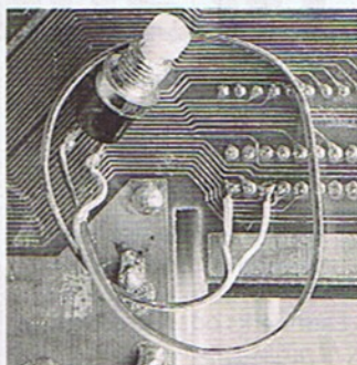
5 Der Reset-Taster am Expansion-Port. Ob Sie den Reset-Taster am User- oder Expansion-Port anschließen, ist gleich.
