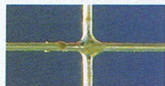
3 So sieht eine richtige Lötstelle aus
