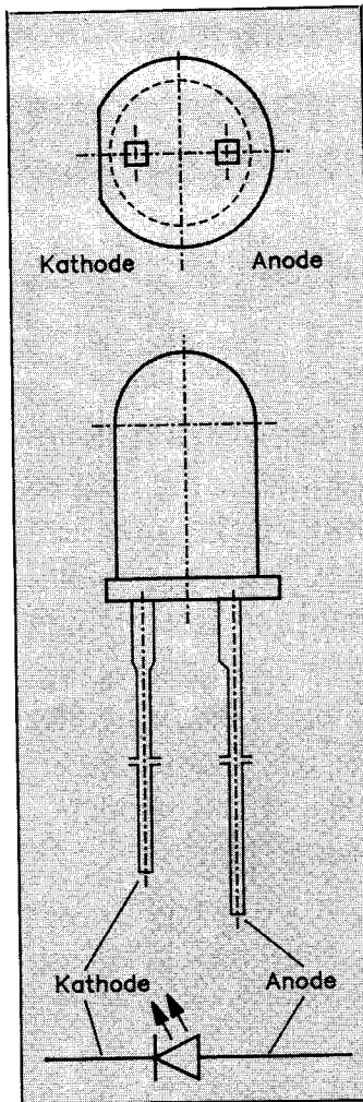
11 Eine Leuchtdiode mit zugehörigem Schaltsymbol. Die Anode einer Leuchtdiode ist meistens dadurch gekennzeichnet, daß das Anschlußbeinchen etwas länger ist.
