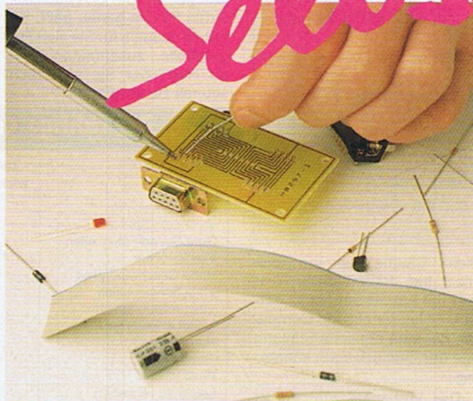
Hier wird gerade eine Joystickbuchse auf die zweite Platine des Tiny-EPROMers gelötet – nicht etwa ein Stecker ...
