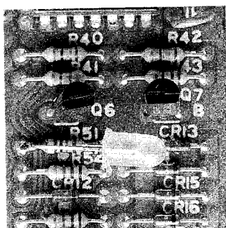
10 Mit geringem Aufwand läßt sich eine optische Schreibkontrolle bei der 1541 realisieren
