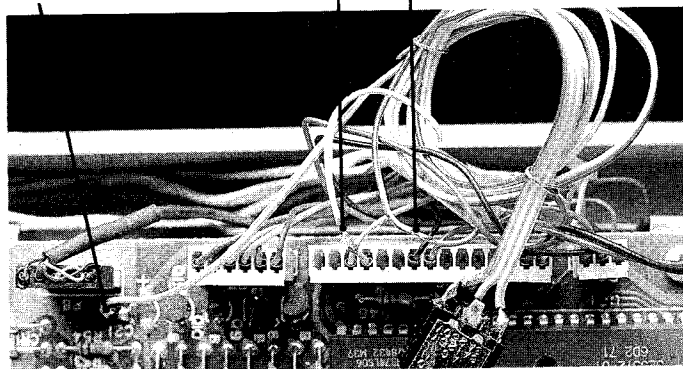
12 So wird der Schalter zur Umgehung der Schreibschutzkennung angeschlossen
