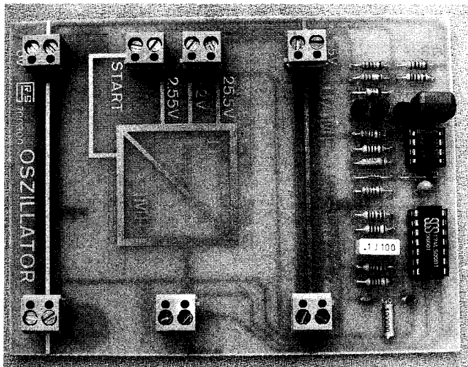
3 Der fertige A/D-Wandler (Bausatz)
