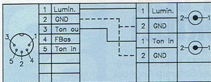
2 So wird ein monochromer Monitor im 40-Zeichen-Modus des C64 oder des C128 angeschlossen
