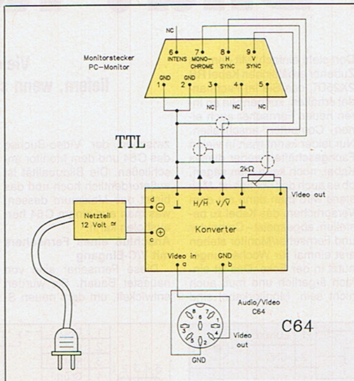
So wird die Platine an den Monitor und Computer angeschlossen
