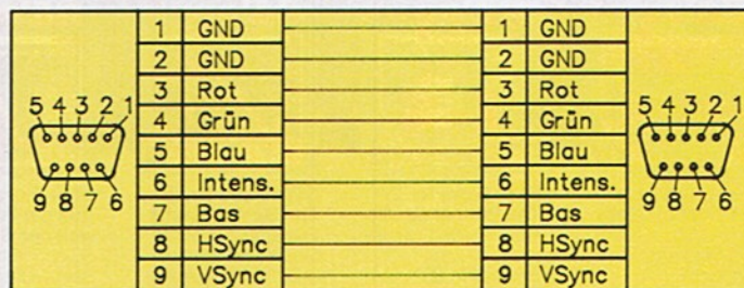
6 Für RGB-Digitalmonitore gilt zum Anschluß an den C128 dieses Schema
