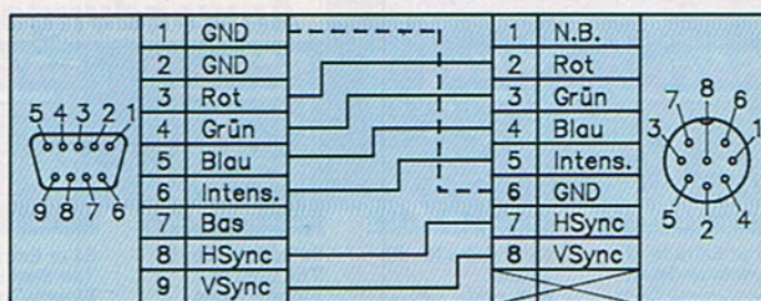
7 Manche RGB-Digitalmonitore besitzen eine achtpolige Anschlußbuchse, dann muß das Kabel so aussehen.
