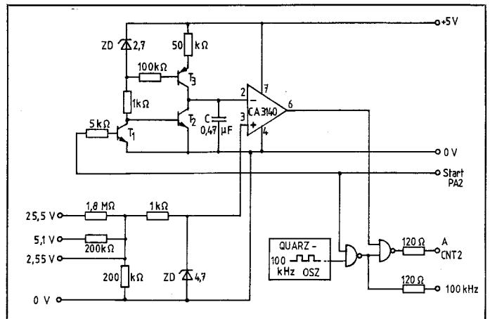
2 Ausführliches Schaltbild des A/D-Wandlers
