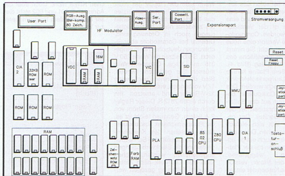
2 Die Platine des C128 D in der Plastikversion ist baugleich mit der normalen 128er Platine, nur der Tastaturanschluß liegt jetzt außen
