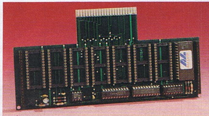
Ein Modul ist die einfachste Art, EPROMs zu verwenden
