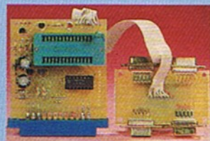
Der Tiny-EPROMer
