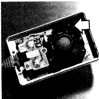
Die geöffnete Maus 1351 - der Pfeil kennzeichnet den Öl-Punkt.
