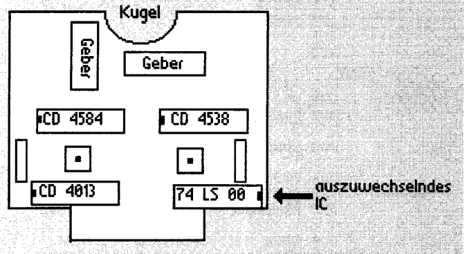
Nach dem IC-Tausch ist Ihre Maus Geos-kompatibel
