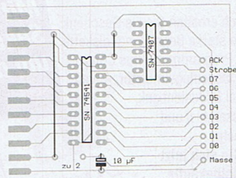
6 Der Bestückungsplan des Leitungstreibers. Mit nur zwei ICs lassen sich Entfernungen bis zu fünf Metern überbrücken
