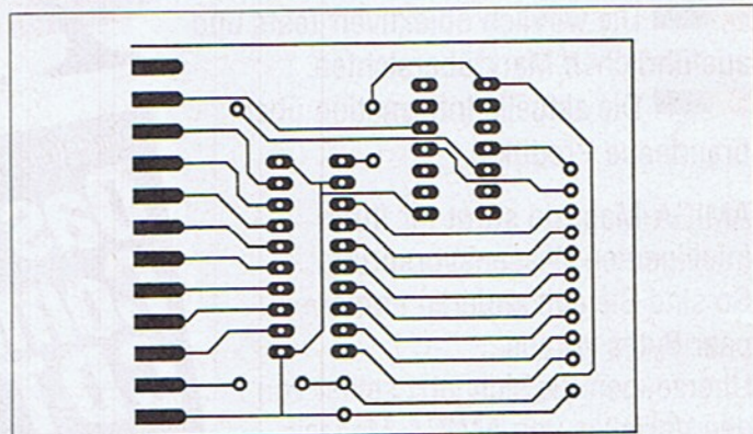
8 Das Layout der Treiberplatine
