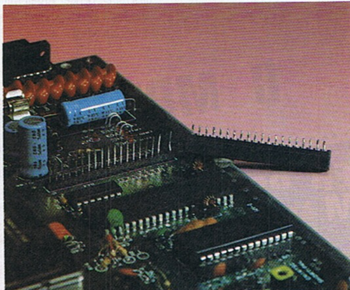
13 Der Tastaturstecker im C64
