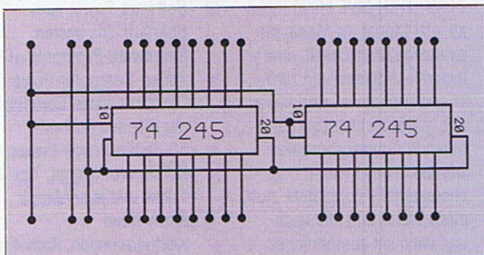
2 Mit zwei ICs ist die CIA sicher geschützt
