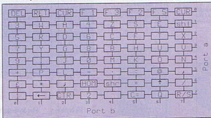
1 Die Tastatur-Matrix des C64
