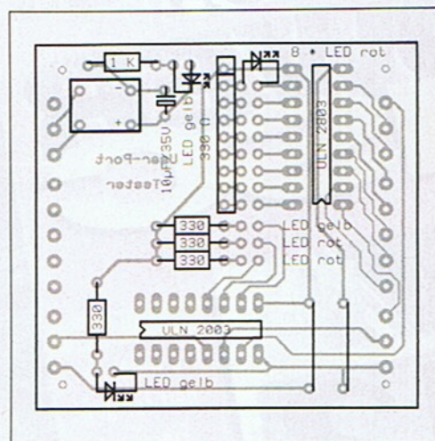
Der Bestückungsplan des Testmoduls. Beachten Sie die richtige Polung des Widerstands-Arrays.
