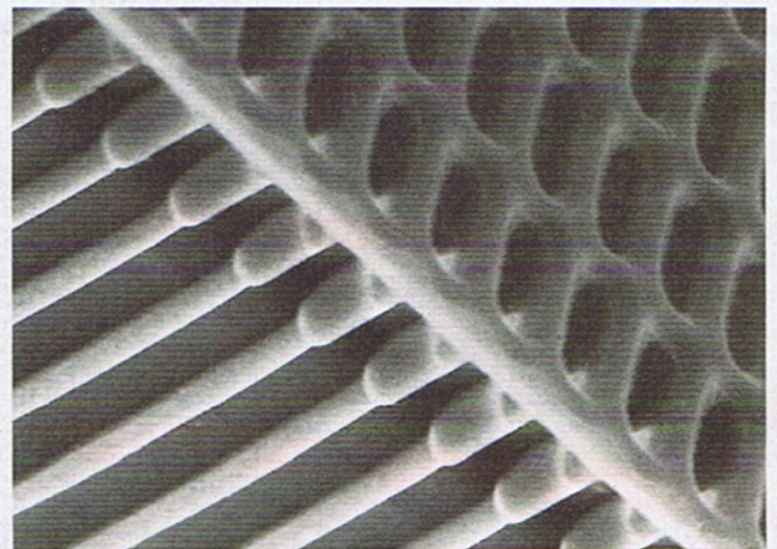
Rasterelektronenaufnahme eines dynamischen Speichers neuester Technologie
