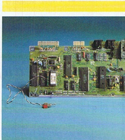
Nun kann eine 28polige Fassung eingesetzt werden. Sie wird unten sorgfältig verlötet. Dann wird die Adapterplatte mit dem neuen EPROM richtig (Kerbe des neuen EPROMs zeigt in Richtung des User-Ports) herum in den C64 gesteckt. Für den Schalter muß hinten im Gehäuse noch ein Loch gebohrt werden. Danach kann der Zusammenbau des C64 in umgekehrter Reihenfolge stattfinden.
