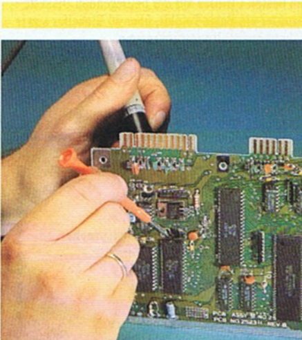
Deshalb hebeln wir den Chip während des Erhitzens mit einem Schraubendreher an einer Seite hoch. Dies wiederholen wir an der gegenüberliegenden Seite, bis der IC unbeschädigt herauskommt.
