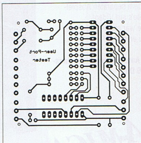
Die Platine des Meßmoduls: Achten Sie auf den richtigen Einbau des Widerstands-Arrays.
