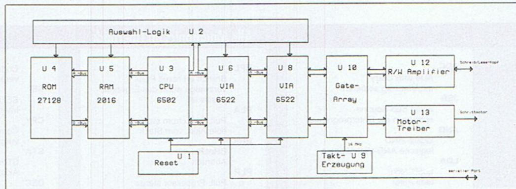
1 Der Blockschaltplan der Elektronik zeigt einen kompletten Computer
