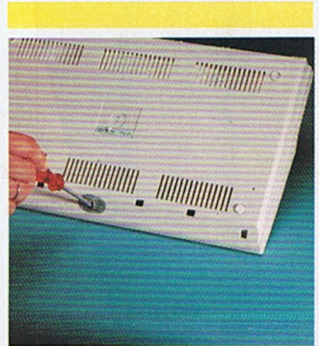
Zuerst wird der C64 geöffnet. Dazu sind entweder die Klammern an seiner Unterseite mit einem Schraubendreher nach außen zu drücken oder drei Schrauben zu lösen. Dabei geht das Garantiesiegel kaputt. (Achtung Garantieverlust!) Das Oberteil mit der Tastatur kann nun abgehoben werden.
