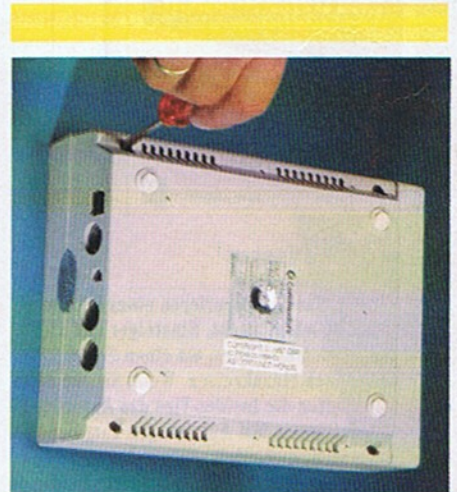
Das Diskettenlaufwerk wird umgedreht und alle vier Schrauben an der Unterseite werden entfernt. Jetzt kann das Laufwerk aus der oberen Halbschale gehoben werden.
