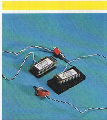
Das Wichtigste: Jiffy-DOS. Es besteht aus zwei EPROMs, eins davon befindet sich auf einer Adapterplatte zum Einbau in den C64, eins wird in die Floppy eingesetzt.
