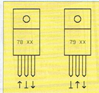
Positive und negative Stabis haben unterschiedliche Anschlußfolgen
