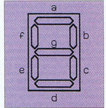
Die LEDs im Display werden mit a bis g bezeichnet
