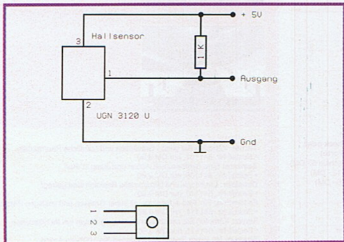
Die Schaltung des Windsensors besteht entweder aus einem Reed-Kontakt oder einem Hallsensor
