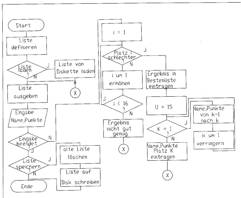
So läuft die Sortierung einer Bestenliste ab
