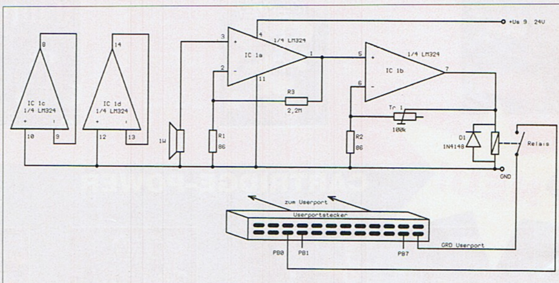
Schaltbild des Akustikrelais: An den Userportstecker müssen nur zwei Leitungen angelötet werden.
