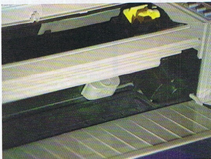
In der Laufschiene des Druckkopfs setzen sich oft Papierschnipsel fest, die die Bewegung behindern
