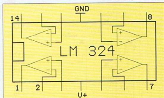
▲ ▼ Anschlußplan LM 324 (o.) und Reedrelais (u.)
