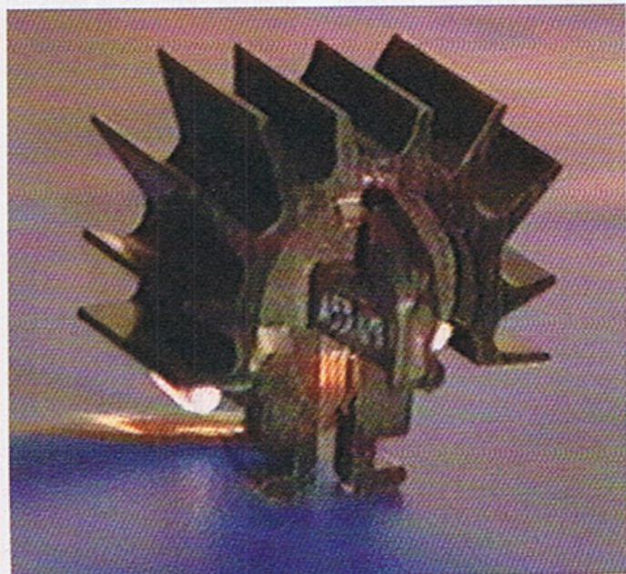
Der Druckkopf eines Nadeldruckers wird im Betrieb sehr heiß. Ein Kühlkörper sorgt für erträgliche Temperaturen.
