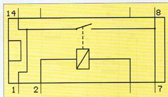
▲ ▼ Anschlußplan LM 324 (o.) und Reedrelais (u.)
