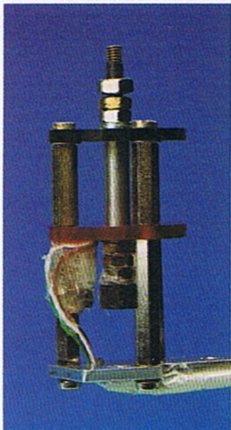
Im Detailfoto erkennt man deutlich den aufgeklebten Hallsensor
