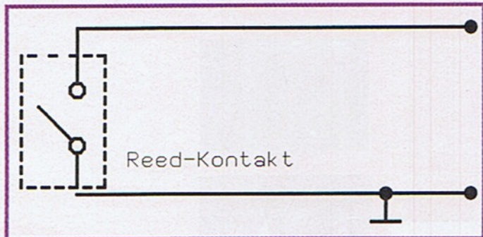
Die Schaltung des Windsensors besteht entweder aus einem Reed-Kontakt oder einem Hallsensor
