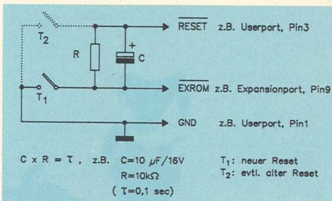
Bild 3. Universeller Reset am Expansion-Port.
