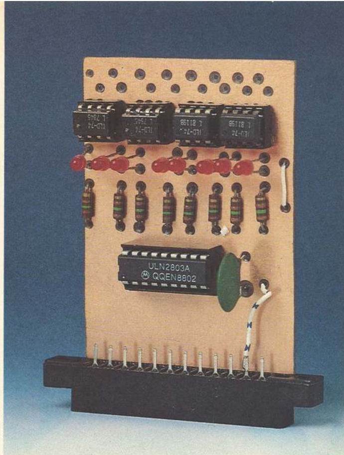
Bild 4. Der Relaistreiber mit Display.
