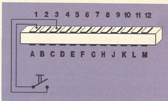
Bild 1. Reset am Userport (von hinten gesehen).
