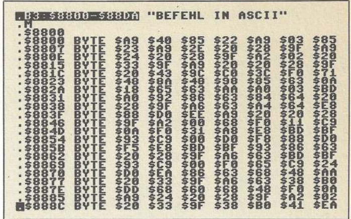
[3] Durch den Befehl ».M« werden alle Speicherinhalte in hexadezimaler Form ausgegeben
