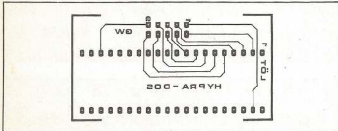
[4] Layout des 40poligen Zwischensockels für das Parallelkabel. Achtung: Das Layout ist spiegelverkehrt im Verhältnis 1:1.
